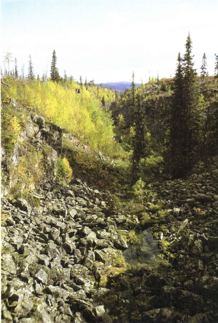
Fig. 31. The proglacial gorge of Nuoluskuru.
